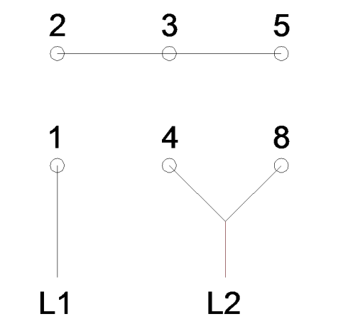
230V MOTOR WIRING
